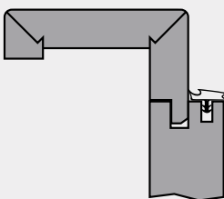
4 ZARGE MIT KLEINER RUNDKANTE FRAME WITH SMALL ROUNDED EDGE
